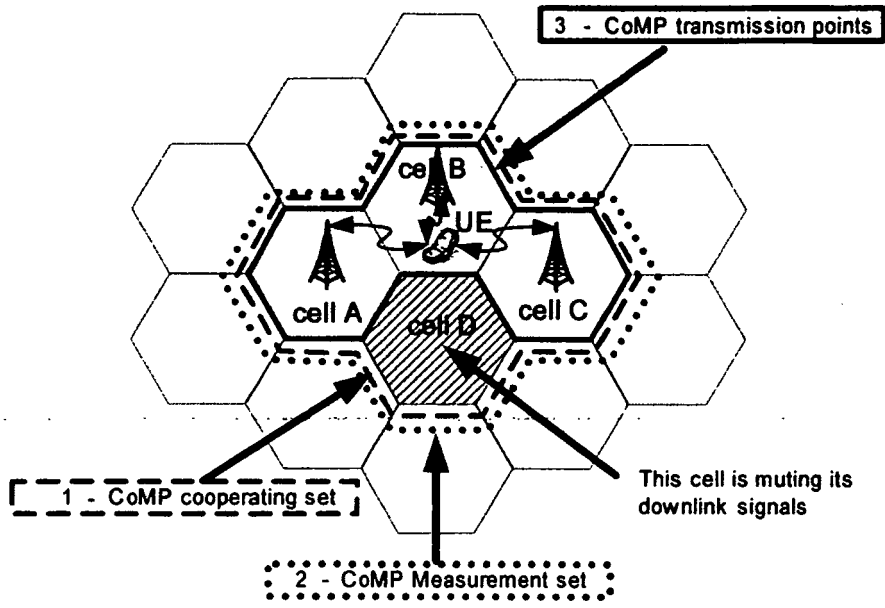
(a) CoMP JP
