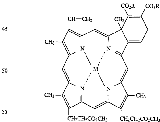
Complex VI
