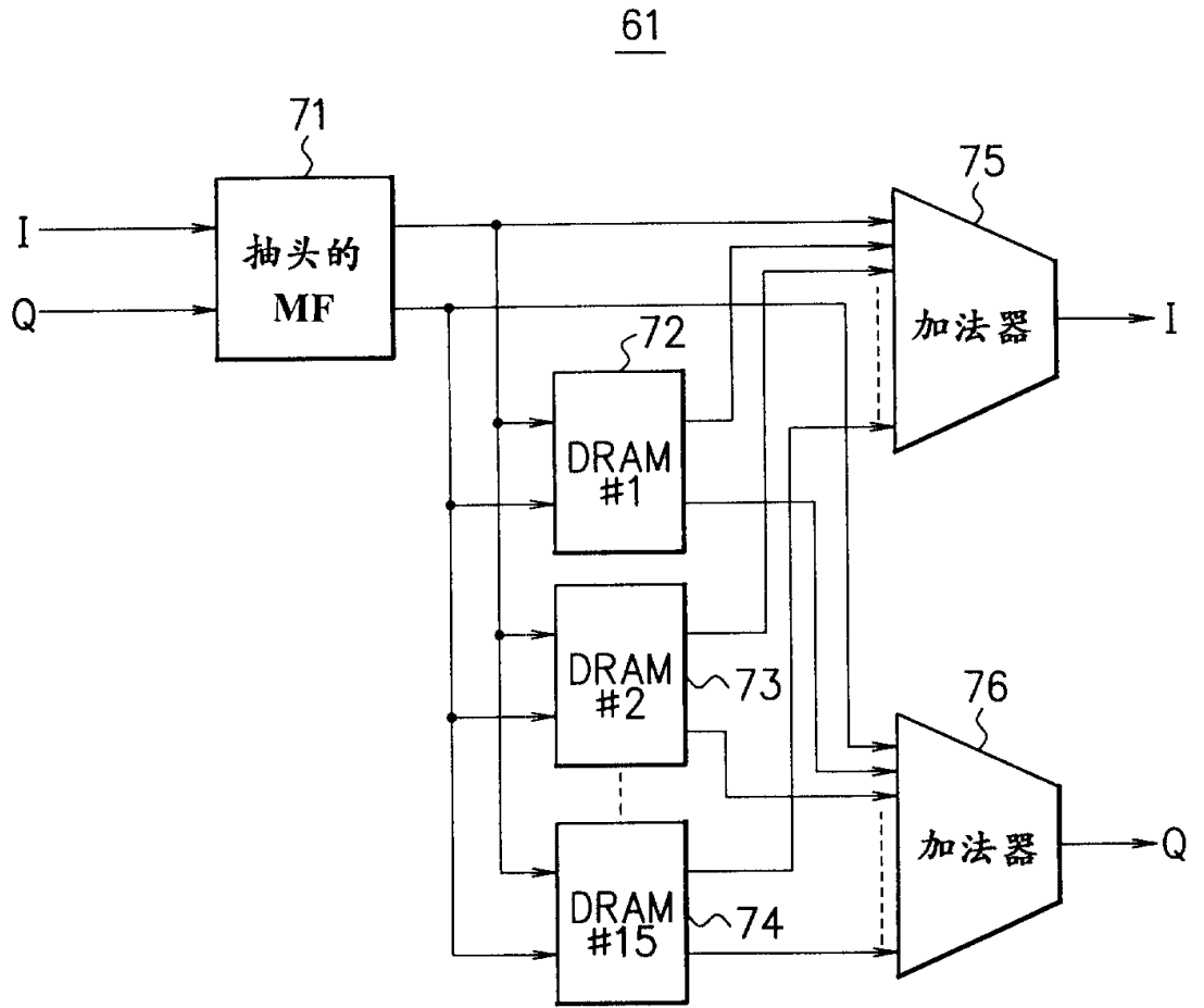
第三实施方式的相关器的框图
