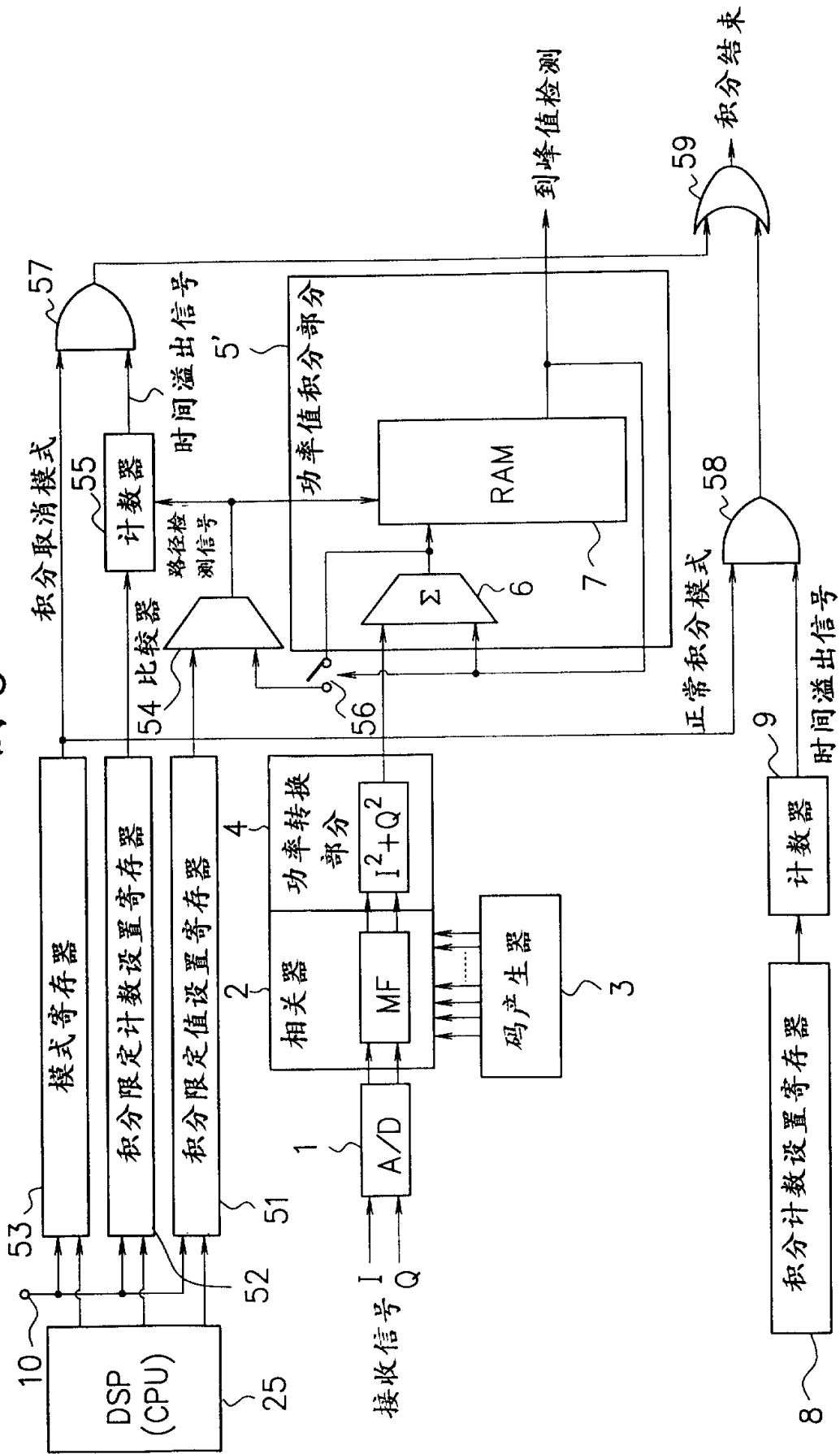
第二实施方式的小区搜寻的框图
