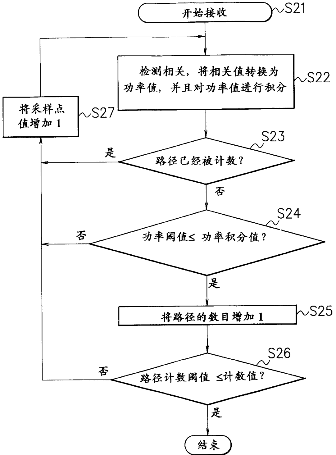
显示第二实施方式的小区搜寻操作的流程图
