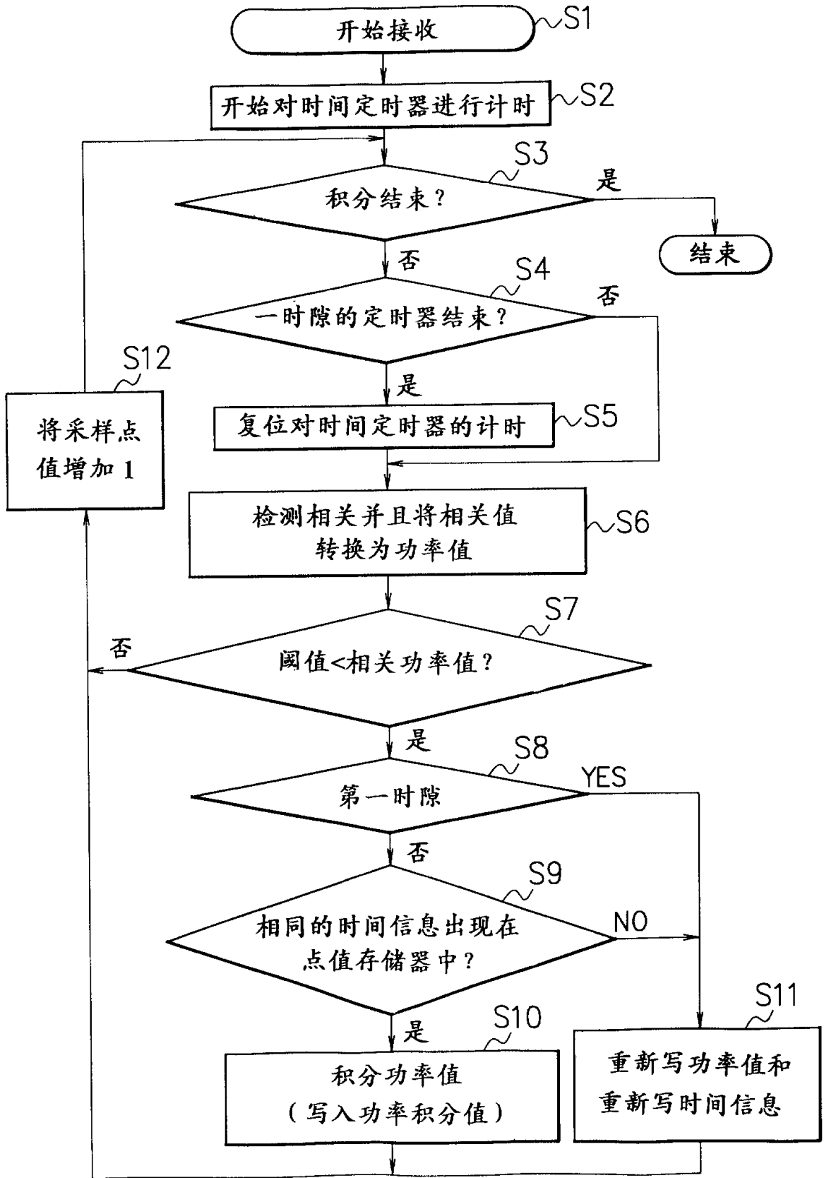
显示第一实施方式的小区搜寻操作的流程图
