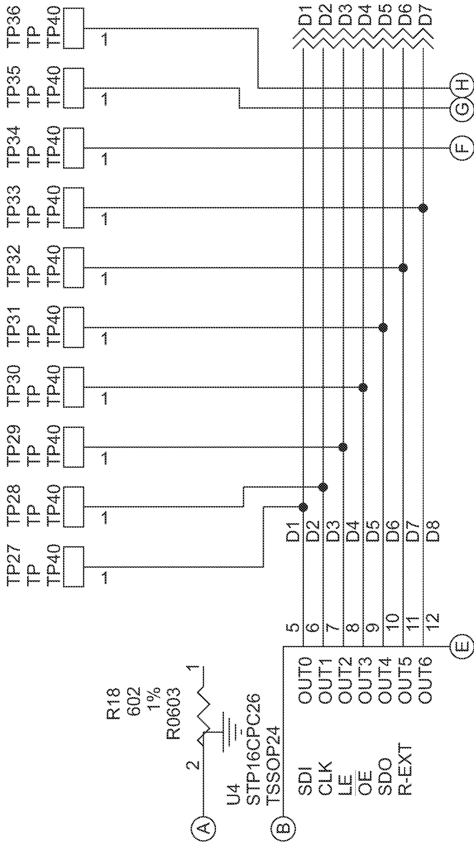
FIG. 10D (Cont'd)
