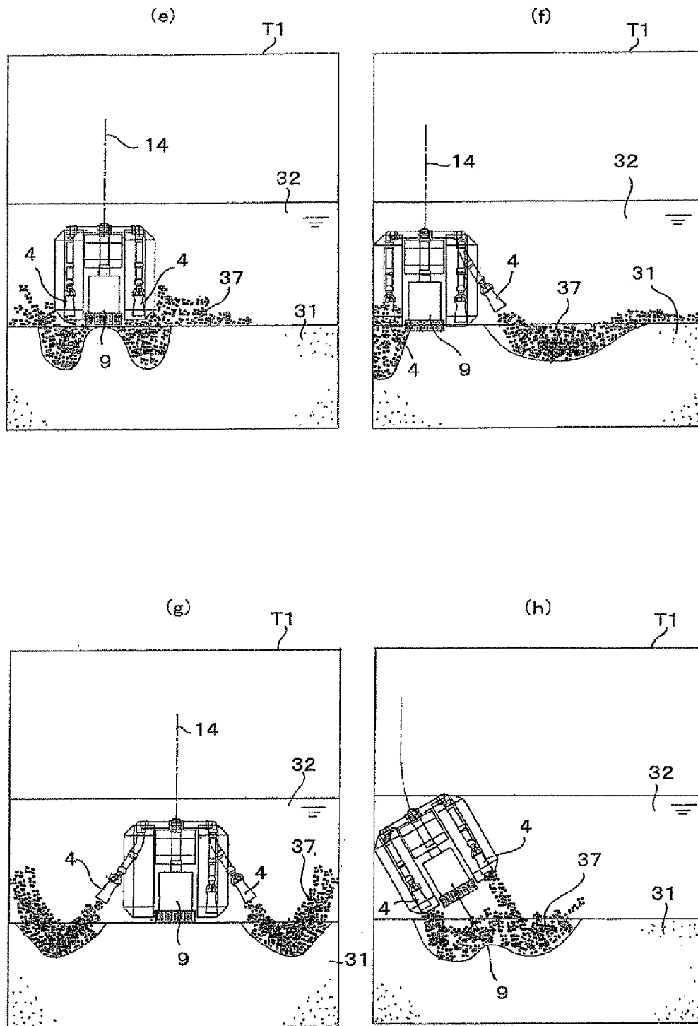
FIG.7(2)
