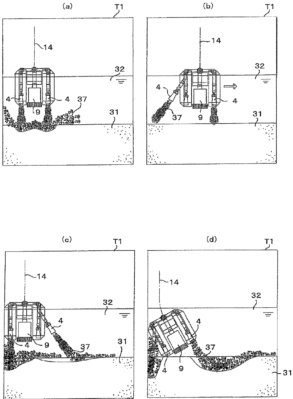
FIG.7(1)
