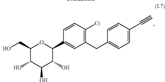
1-chloro-4-(β-D-glucopyranos-1-yl)-2-(4-ethynyl-benzyl)-benzene
