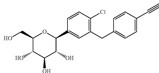
1-chloro-4-(β-D-glucopyranos-1-yl)-2-(4-ethynylbenzyl)benzene
