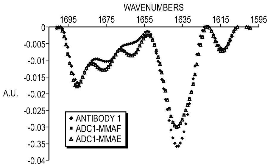
FTIR FIG. 4A
