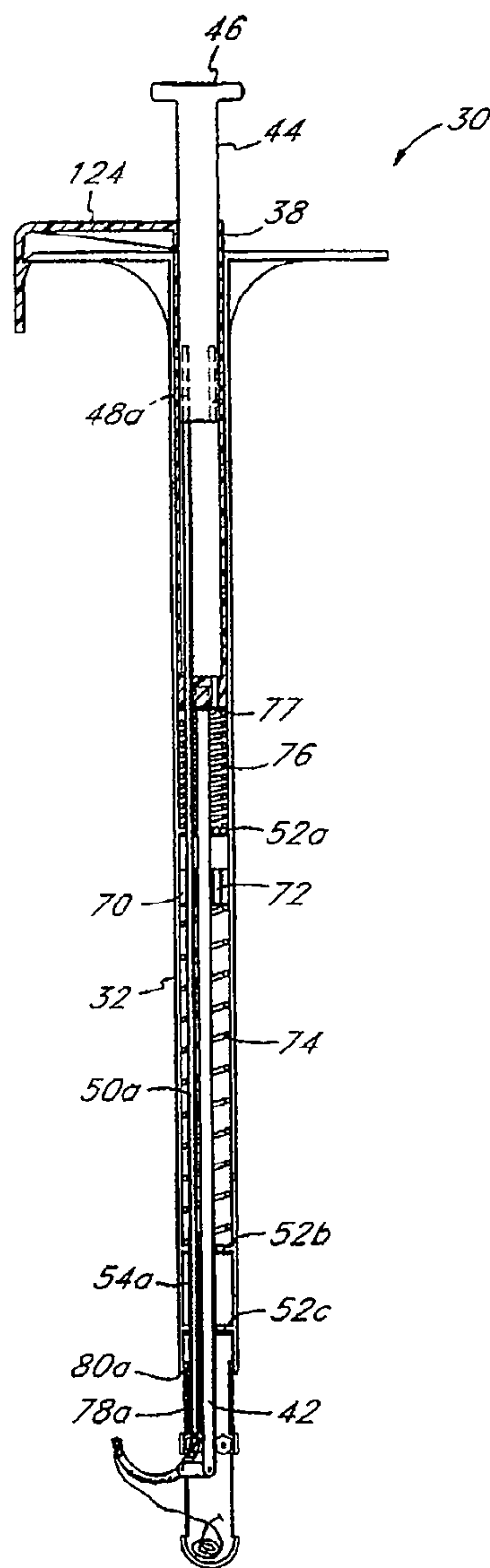
FIG. 3b
