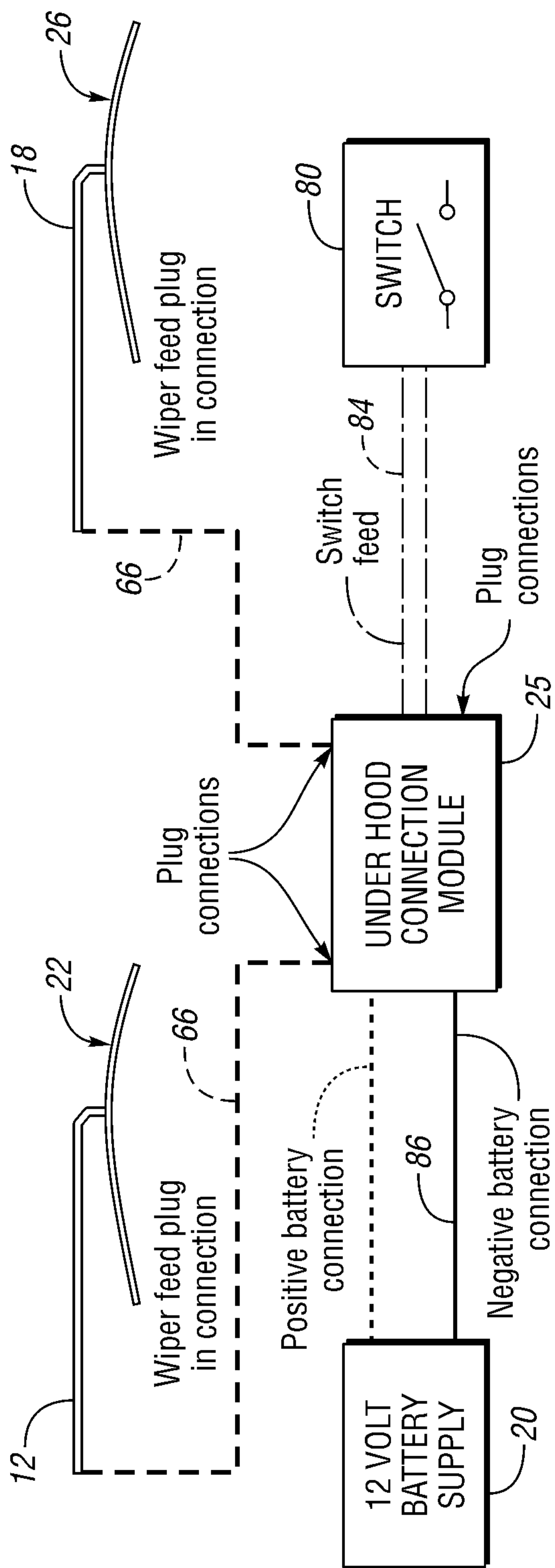
Fig. 6
