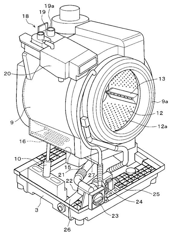
12: 洗い槽 22: 抗菌剤 16: 温水ヒータ 24: 循環ポンプ 21、27: 循環経路
