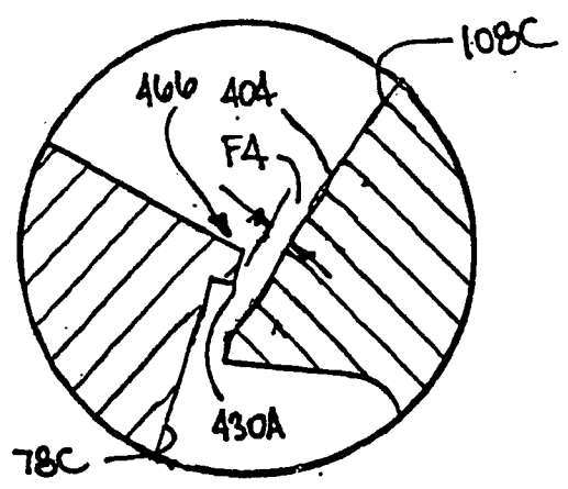
FIG. 16D
