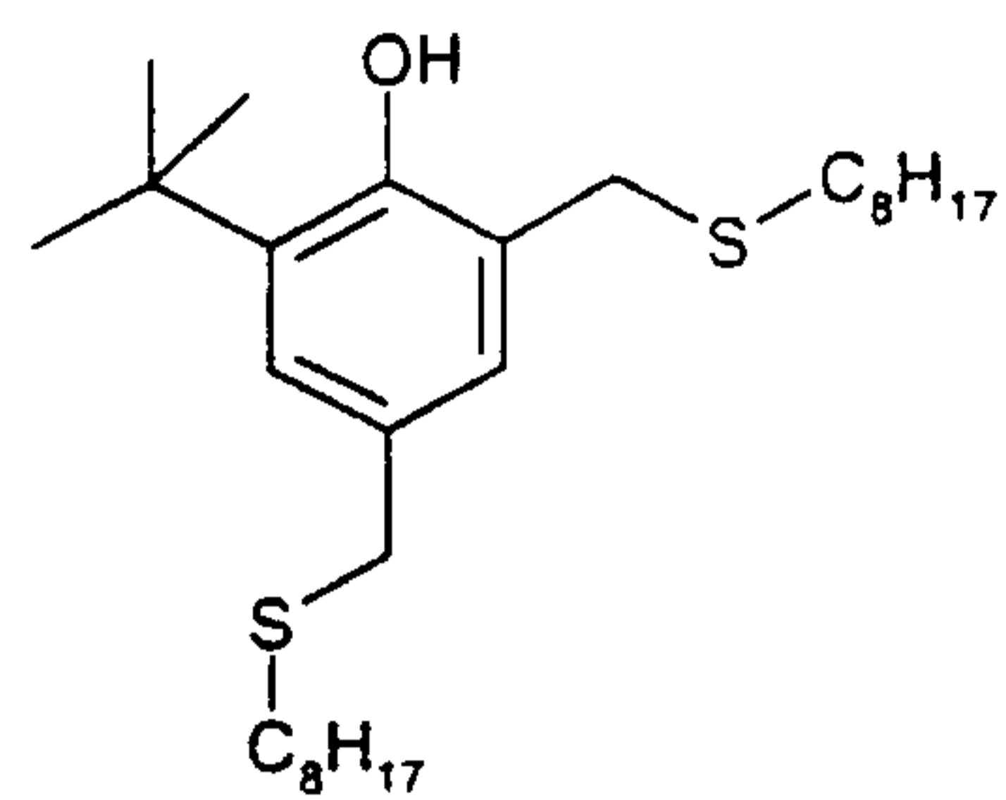
9 IRGANOX 1520
