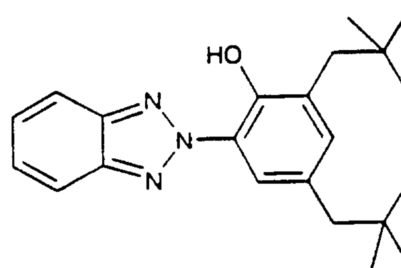
32 TINUVIN 328
