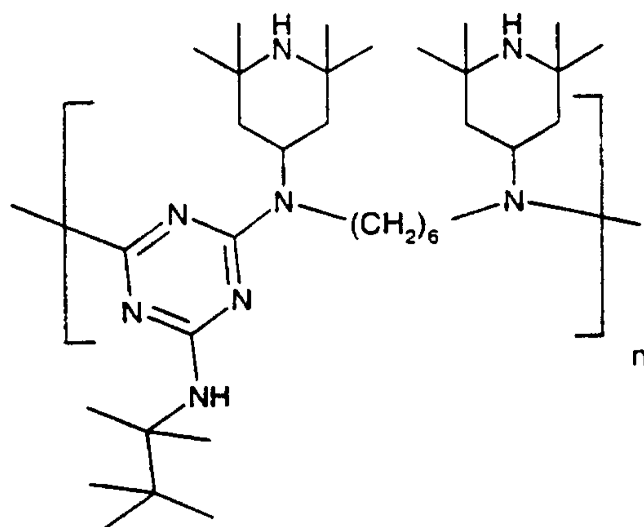
25 CHIMASSORB 944
