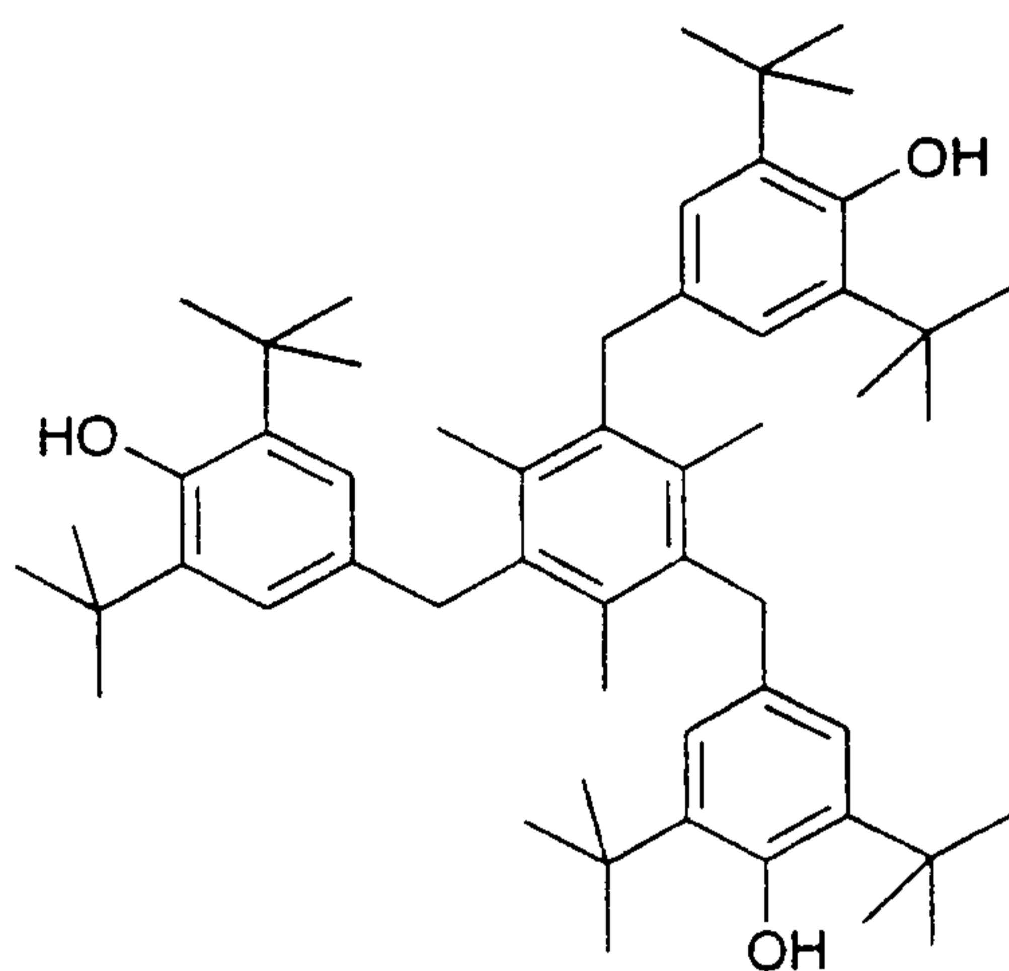
10 IRGANOX 1330
