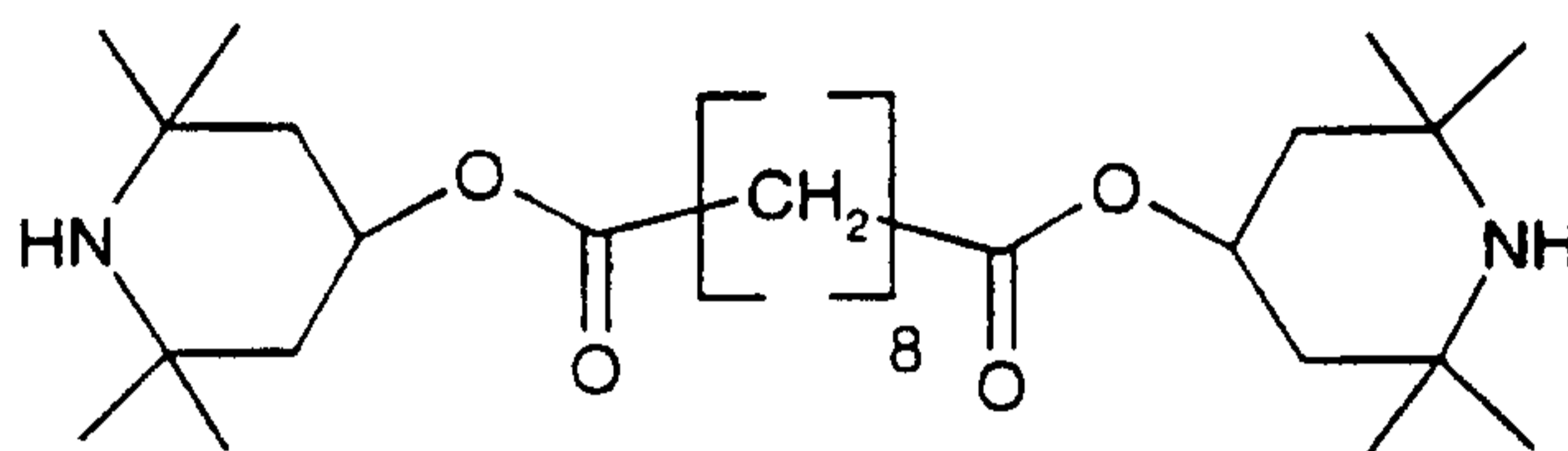
21 TINUVIN 765
