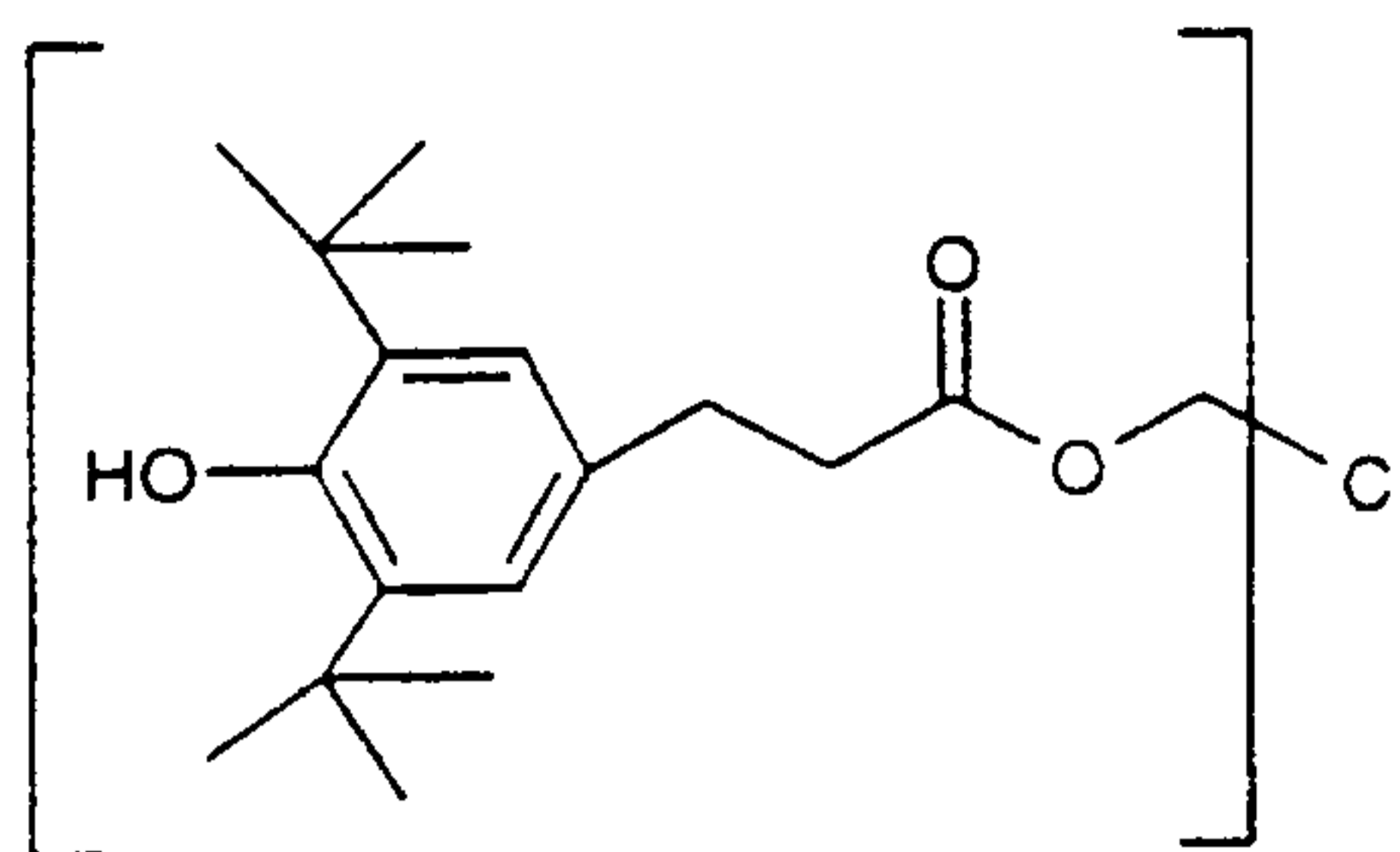
8 IRGANOX 1010
