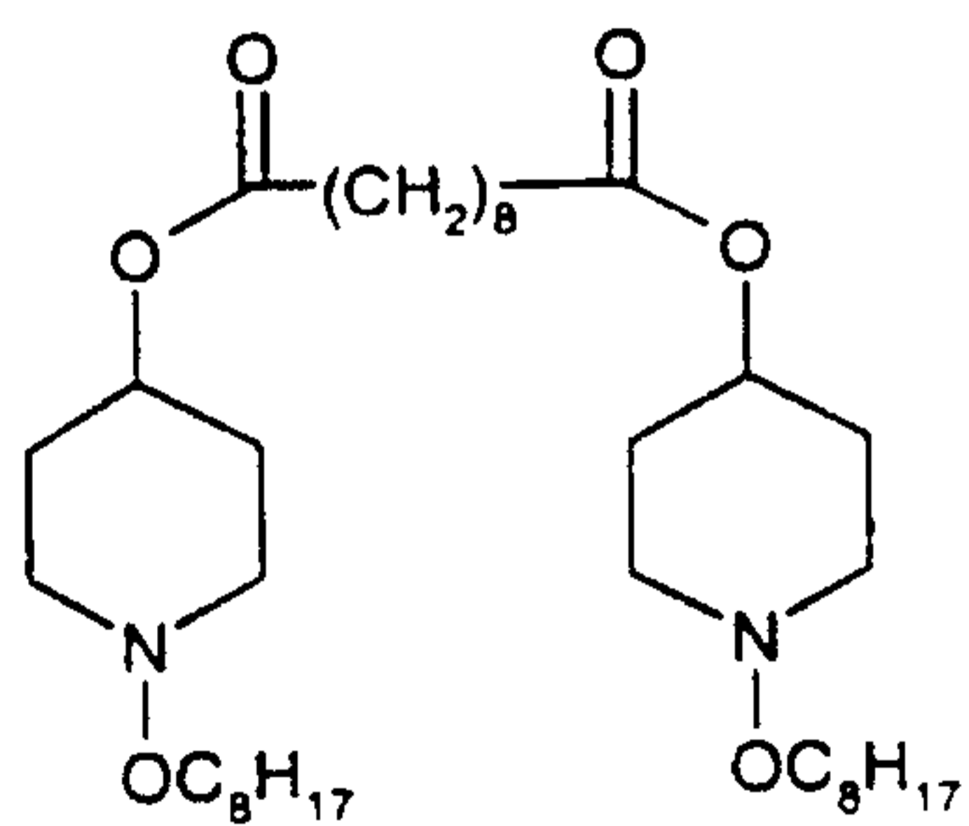
31 TINUVIN 123
