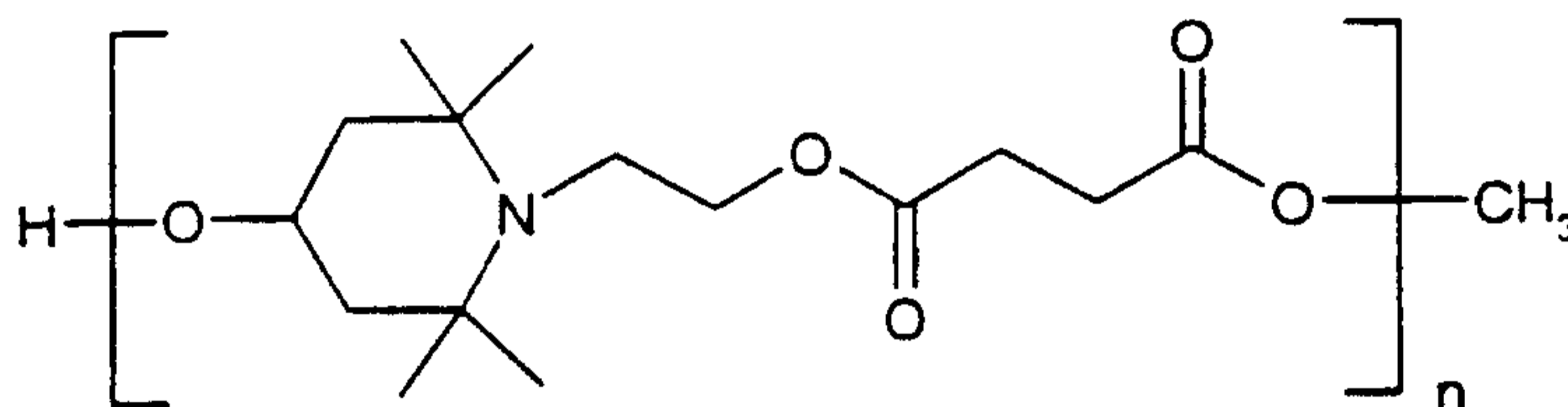
23 TINUVIN 622
