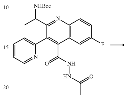
tert-Butyl 1-(4-(2-acetylhydrazinecarbonyl)-6-fluoro-3-(pyridin-2-yl)quinolin-2-yl)ethylcarbamate
