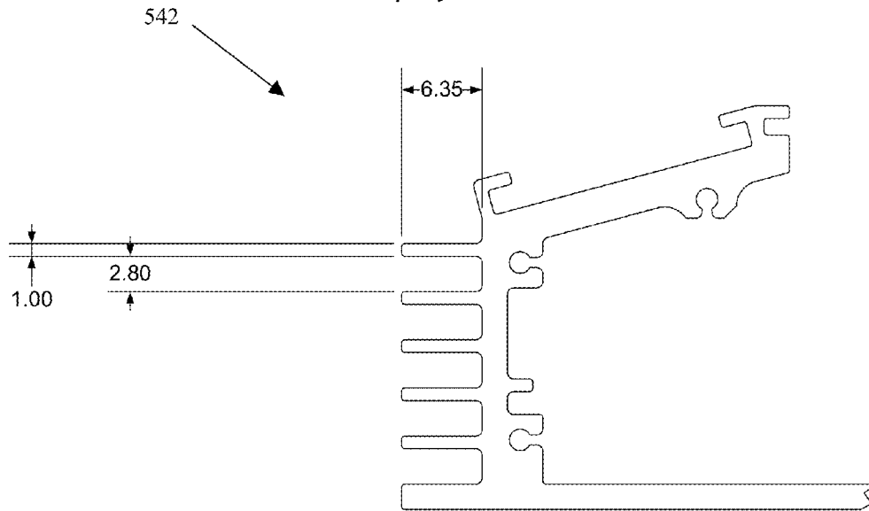
FIG. 3A Exemplary extrusion fin dimensions in mm
