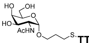
Tn-TT conjugate
