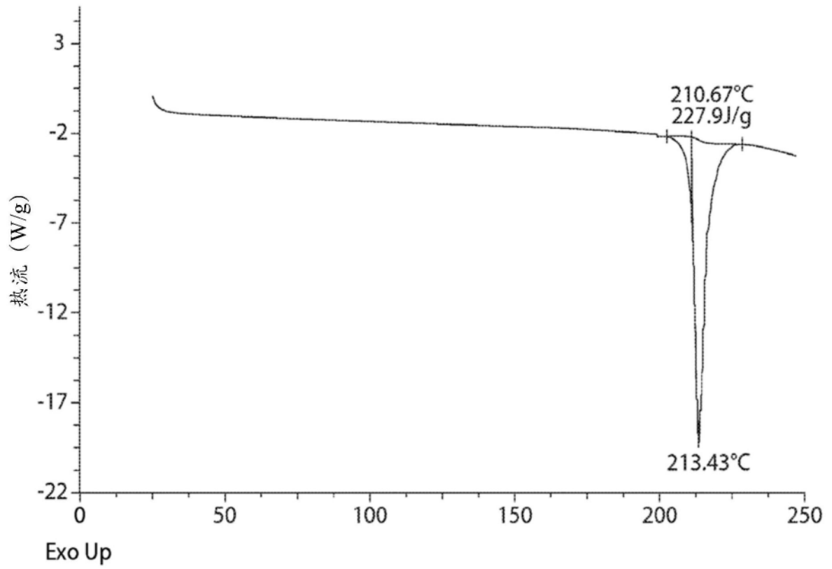
温度 (°C) 形式 3 的 DSC 曲线
