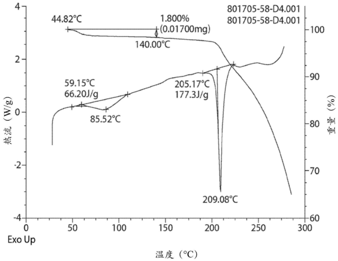
形式4的DSC和TGA曲线
