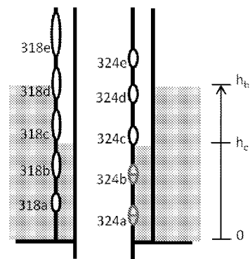
(d) Case 3 SSS outlet riser discharge
