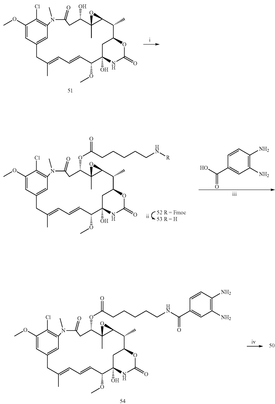
Scheme V-4.
