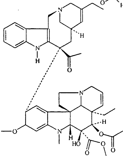
Vinorelbine
