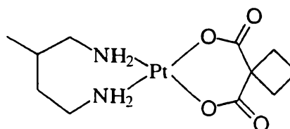
CI-973
