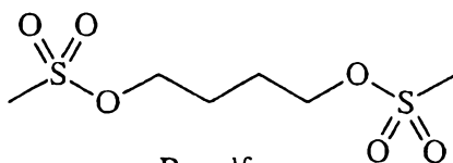
Busulfan
