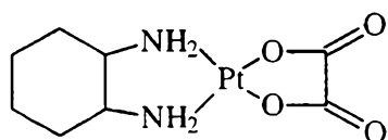
Oxaliplatin
