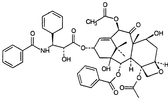
Taxol
