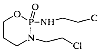
Ifosfamide
