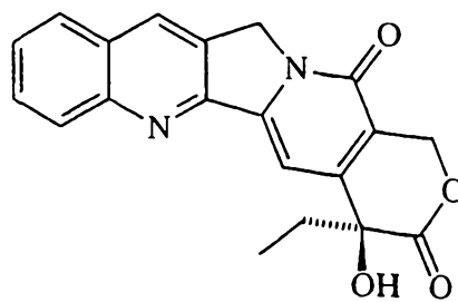
Camptothecin
