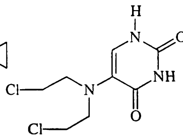
Uracil Mustard
