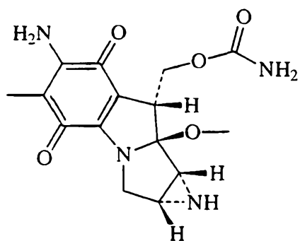
Mitomycin
