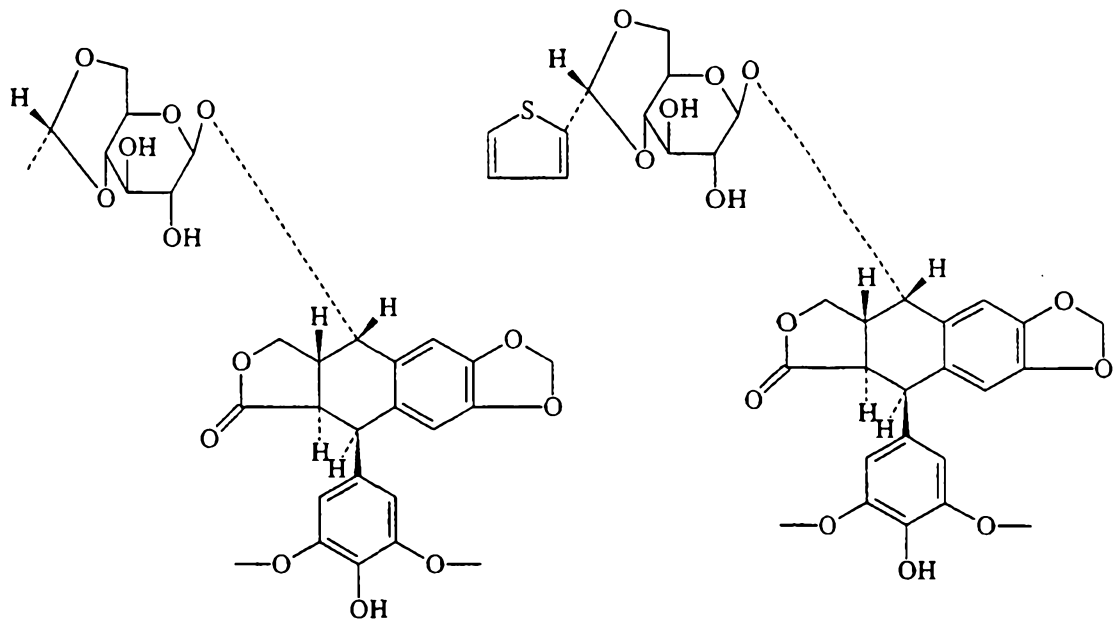
Etoposide
