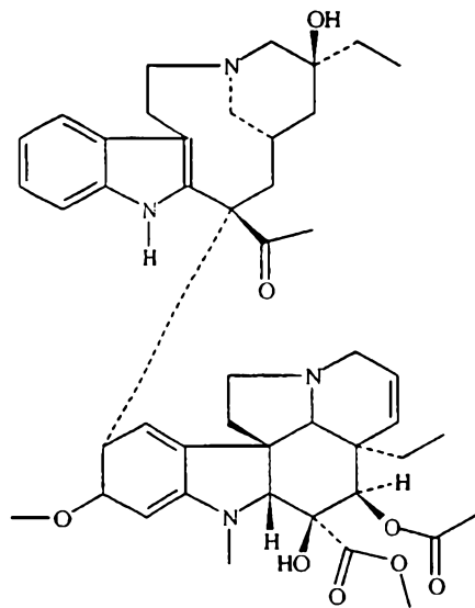
Vinblastine
