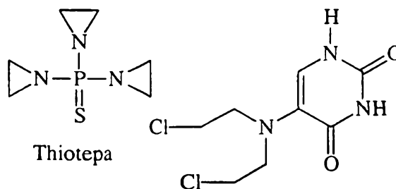
Uracil Mustard
