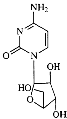
Cytarabine
