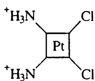
Cisplatin
