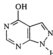
Allopurinol
