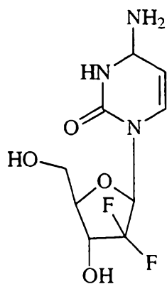
Gemcitabine
