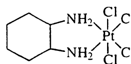
Tetraplatin (Ormaplatin)
