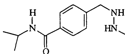
Procarbazine
