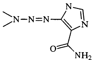
Dacarbazine
