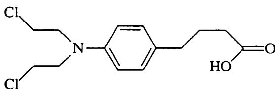
Chlorambucil
