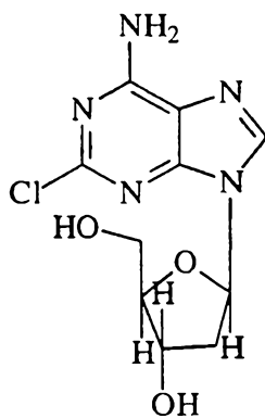
Cladribine
