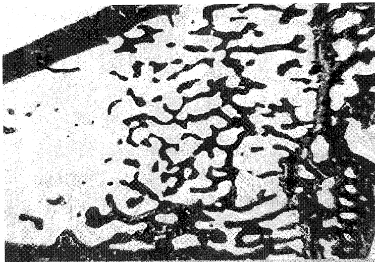
Estradiol + SB-262470
