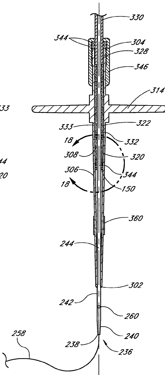
FIG. 17A
