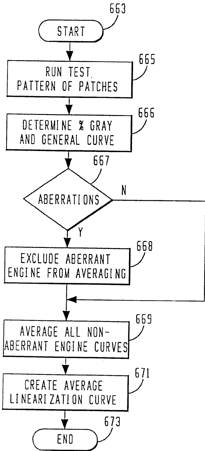
FIG. 33
