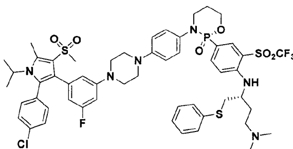
(S)-3-(4-(4-(3-(2-(4-chlorophenyl)-1-isopropyl-5-methyl-4-(methylsulfonyl)-1H-pyrrol-3-yl)-5-fluorophenyl)piperazin-1-yl)phenyl)-2-(4-(((R)-4-(dimethylamino)-1-(phenylthio)butan-2-yl)amino)-3-((trifluoromethyl)sulfonyl)phenyl)-1,3,2-oxazaphosphinane 2-oxide
