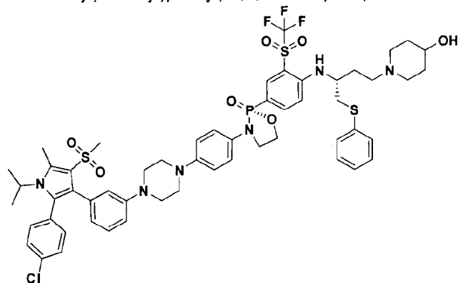
(R)-3-(4-(4-(3-(2-(4-chlorophenyl)-1-isopropyl-5-methyl-4-(methylsulfonyl)-1H-pyrrol-3-yl)phenyl)piperazin-1-yl)phenyl)-2-(4-(((R)-4-(4-hydroxypiperidin-1-yl)-1-(phenylthio)butan-2-yl)amino)-3-((trifluoromethyl)sulfonyl)phenyl)-1,3,2-oxazaphospholidine 2-oxide
