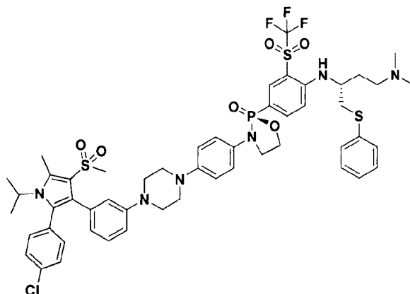
(S)-3-(4-(4-(3-(2-(4-chlorophenyl)-1-isopropyl-5-methyl-4-(methylsulfonyl)-1H-pyrrol-3-yl)phenyl)piperazin-1-yl)phenyl)-2-(4-(((R)-4-(dimethylamino)-1-(phenylthio)butan-2-yl)amino)-3-((trifluoromethyl)sulfonyl)phenyl)-1,3,2-oxazaphospholidine 2-oxide
