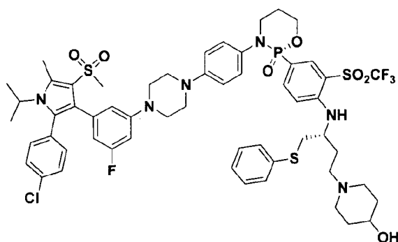
(S)-3-(4-(4-(3-(2-(4-chlorophenyl)-1-isopropyl-5-methyl-4-(methylsulfonyl)-1H-pyrrol-3-yl)-5-fluorophenyl)piperazin-1-yl)phenyl)-2-(4-(((R)-4-(4-hydroxypiperidin-1-yl)-1-(phenylthio)butan-2-yl)amino)-3-((trifluoromethyl)sulfonyl)phenyl)-1,3,2-oxazaphosphinane 2-oxide
