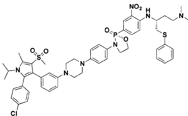
(R)-3-(4-(4-(3-(2-(4-chlorophenyl)-1-isopropyl-5-methyl-4-(methylsulfonyl)-1H-pyrrol-3-yl)phenyl)piperazin-1-yl)phenyl)-2-(4-(((R)-4-(dimethylamino)-1-(phenylthio)butan-2-yl)amino)-3-nitrophenyl)-1,3,2-oxazaphospholidine 2-oxide
