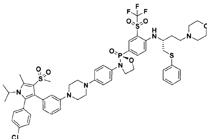
(S)-3-(4-(4-(3-(2-(4-chlorophenyl)-1-isopropyl-5-methyl-4-(methylsulfonyl)-1H-pyrrol-3-yl)phenyl)piperazin-1-yl)phenyl)-2-(4-(((R)-4-morpholino-1-(phenylthio)butan-2-yl)amino)-3-((trifluoromethyl)sulfonyl)phenyl)-1,3,2-oxazaphospholidine 2-oxide
