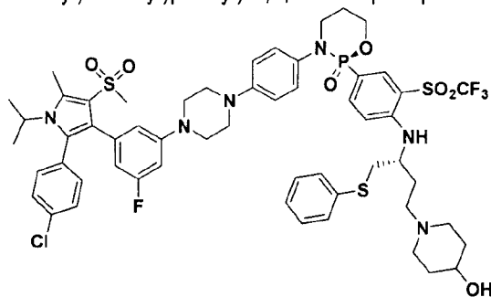
(R)-3-(4-(4-(3-(2-(4-chlorophenyl)-1-isopropyl-5-methyl-4-(methylsulfonyl)-1H-pyrrol-3-yl)-5-fluorophenyl)piperazin-1-yl)phenyl)-2-(4-(((R)-4-(4-hydroxypiperidin-1-yl)-1-(phenylthio)butan-2-yl)amino)-3-((trifluoromethyl)sulfonyl)phenyl)-1,3,2-oxazaphosphinane 2-oxide
