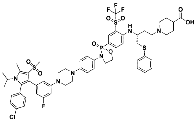
1-((R)-3-((4-((R)-3-(4-(4-(3-(2-(4-chlorophenyl)-1-isopropyl-5-methyl-4-(methylsulfonyl)-1H-pyrrol-3-yl)-5-fluorophenyl)piperazin-1-yl)phenyl)-2-oxido-1,3,2-oxazaphospholidin-2-yl)-2-((trifluoromethyl)sulfonyl)phenyl)amino)-4-(phenylthio)butyl)piperidine-4-carboxylic acid
