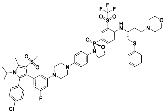
(S)-3-(4-(4-(3-(2-(4-chlorophenyl)-1-isopropyl-5-methyl-4-(methylsulfonyl)-1H-pyrrol-3-yl)-5-fluorophenyl)piperazin-1-yl)phenyl)-2-(4-(((R)-4-morpholino-1-(phenylthio)butan-2-yl)amino)-3-((trifluoromethyl)sulfonyl)phenyl)-1,3,2-oxazaphospholidine 2-oxide
