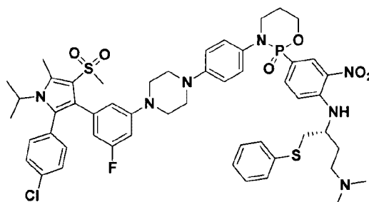
3-(4-(4-(3-(2-(4-chlorophenyl)-1-isopropyl-5-methyl-4-(methylsulfonyl)-1H-pyrrol-3-yl)-5-fluorophenyl)piperazin-1-yl)phenyl)-2-(4-(((R)-4-(dimethylamino)-1-(phenylthio)butan-2-yl)amino)-3-nitrophenyl)-1,3,2-oxazaphosphinane 2-oxide
