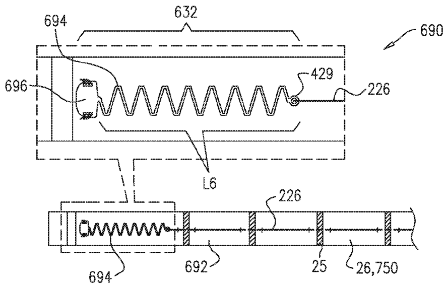
FIG. 29B
