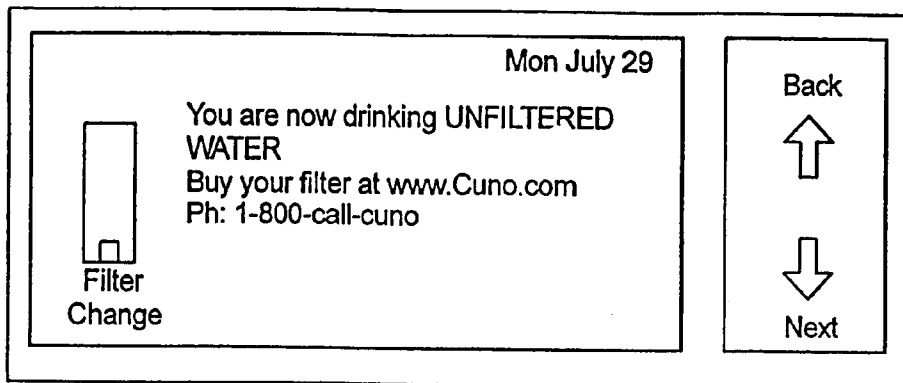
Message Page
