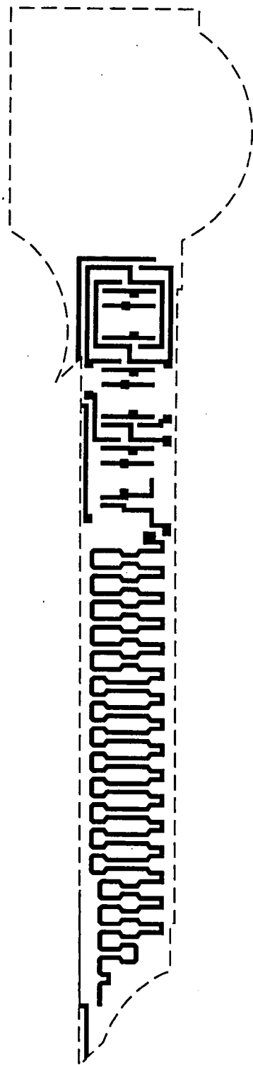
Poly mask
