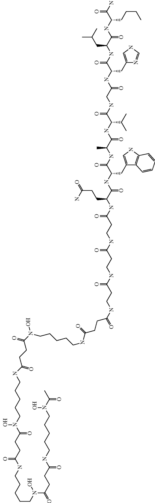
(Ligand III)
