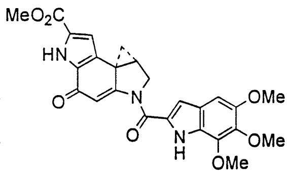
(+)-Duocarmycin SA 3
