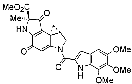
(+)-Duocarmycin A 2
