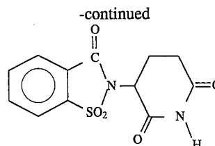
supidimide.
