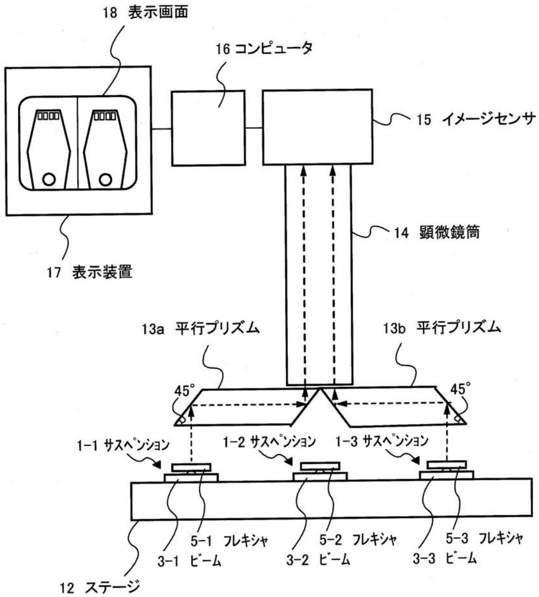
10 測定装置
