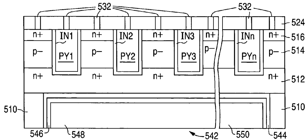
FIG. 5G
