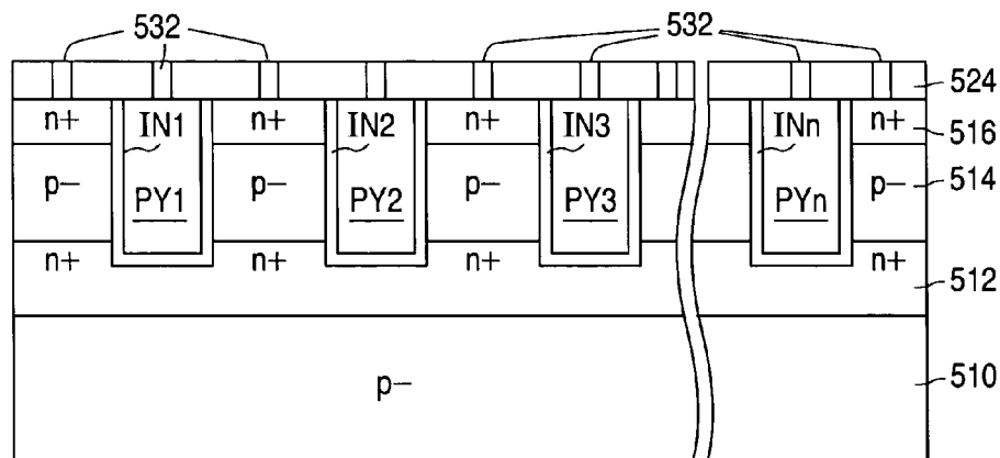
FIG. 5E
