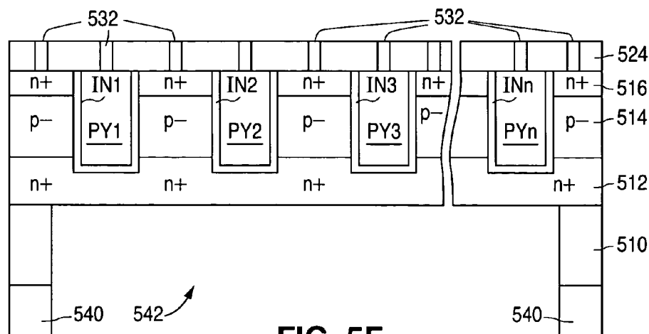
FIG. 5F
