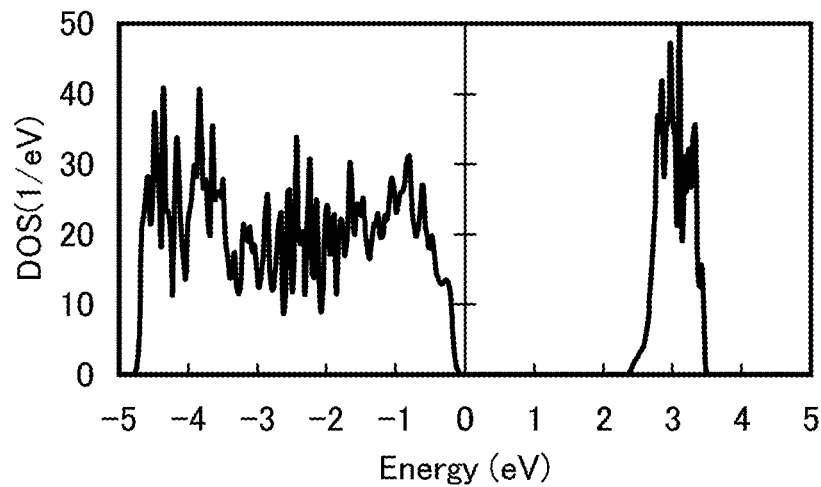
FIG. 12C TiO 2 (Brookite type)
