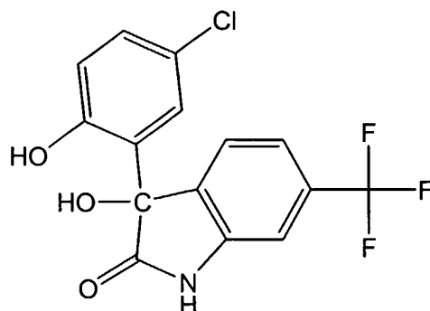
(±)-3-(5-Chloro-2-hydroxyphenyl)-1,3-dihydro-3-hydroxy-6-(trifluoromethyl)-2H-indol-2-one;
