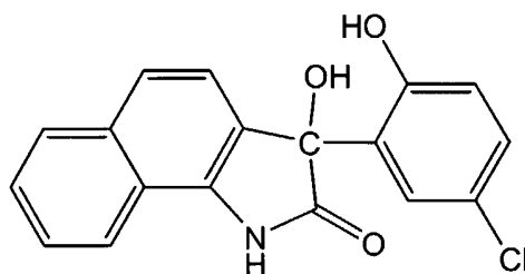
5 (±)-3-(5-Chloro-2-hydroxyphenyl)-1,3-dihydro-3-hydroxy-2H-benz[g]indol-2-one;
