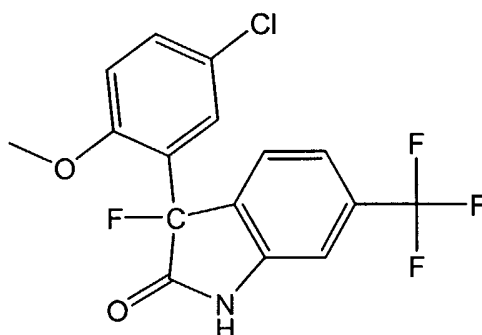
(±)-3-(5-Chloro-2-methoxyphenyl)-1,3-dihydro-3-fluoro-6-(trifluoromethyl)-2H-indol-2-one;
