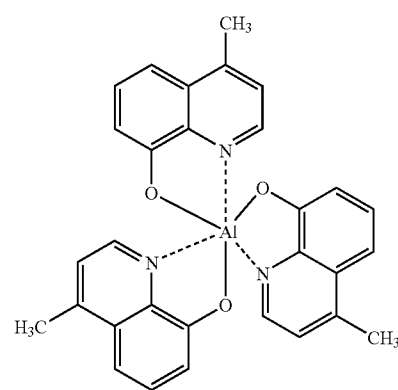
Almq 3
