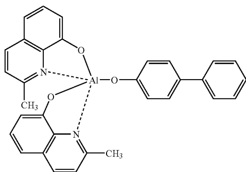
BAlq
