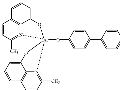
BAlq
