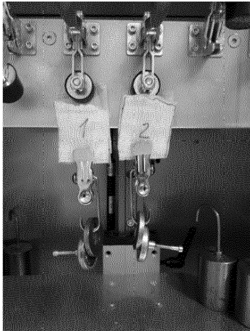
FIG.19B
