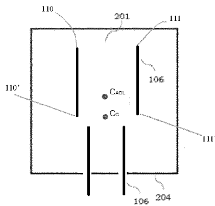
FIG. 17G
