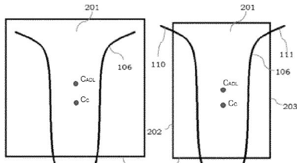
FIG. 17E
