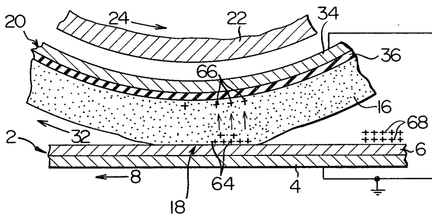
FIG. 3-A PRIOR ART
