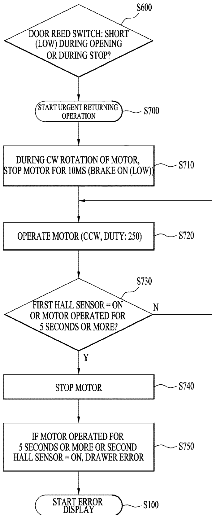
FIG. 36
