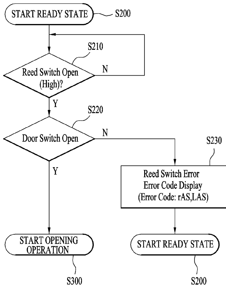
FIG. 32
