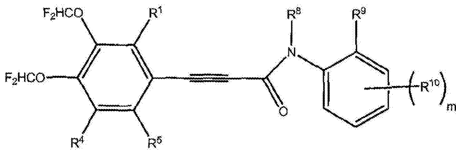
式 (V)
