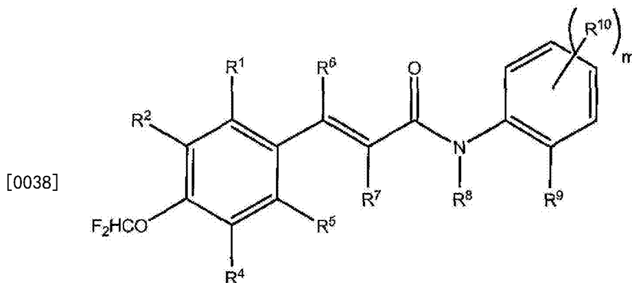
式 (III)
