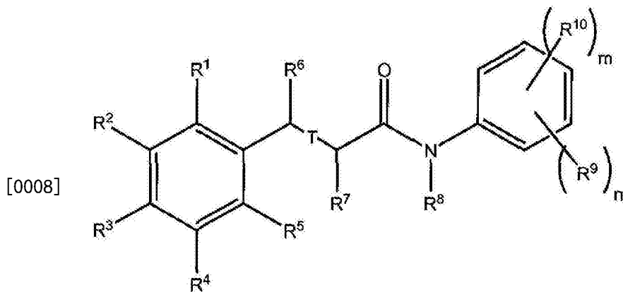
式 (I)
