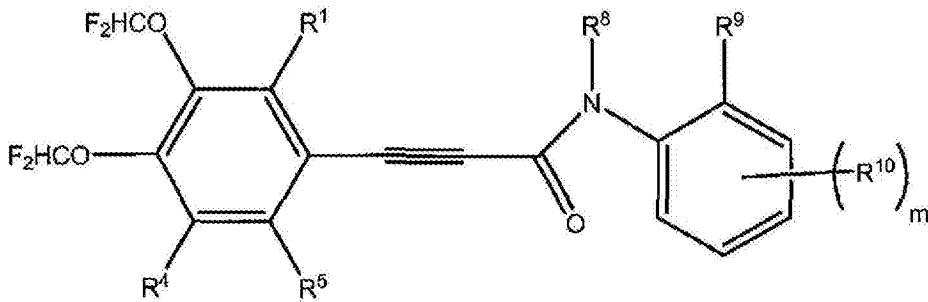
式 (V)
