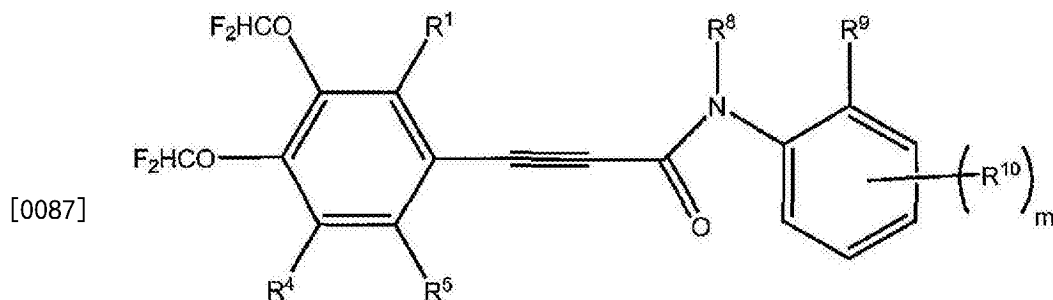
式(V)
