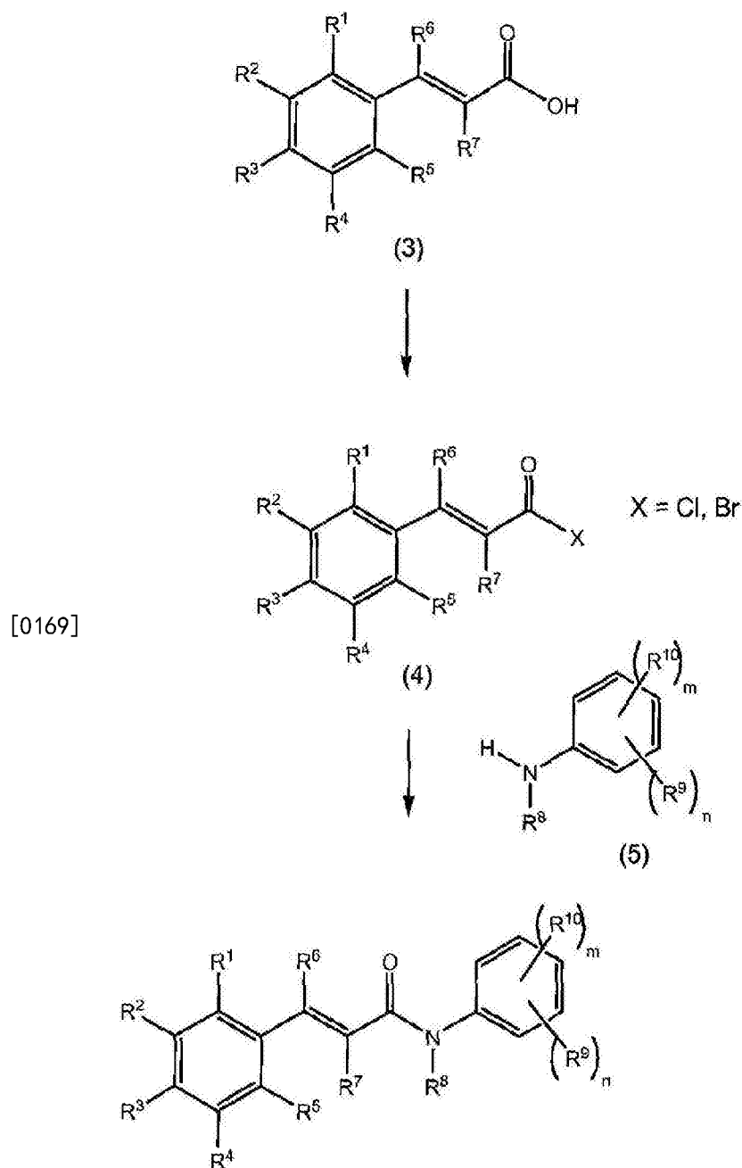
方案 2
