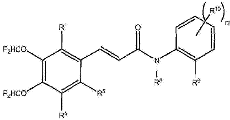
式 (IV)
