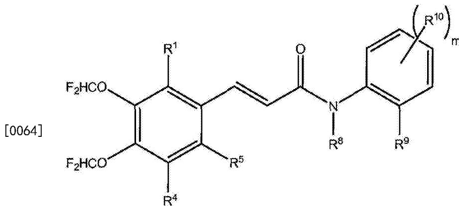
式 (IV)
