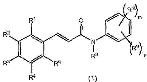
方案 1
