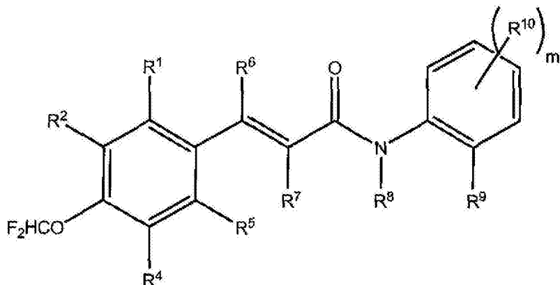
式(III)
