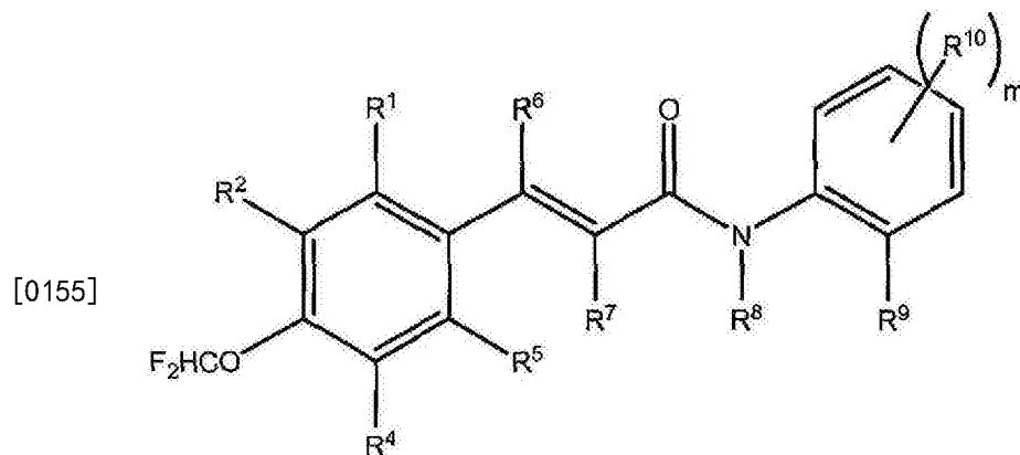
式 (III)
