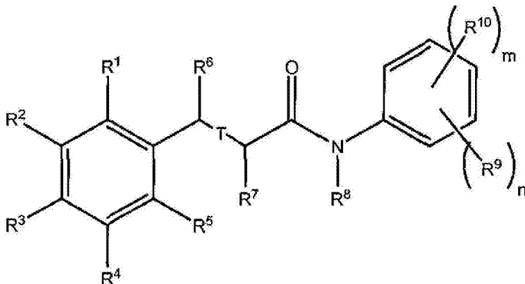
式 (I)
