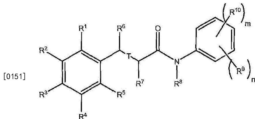
式 (I)
