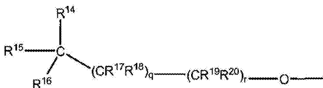
式 (II)
