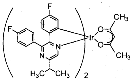
Ir(Fdppr-iPr) 2 (acac)
