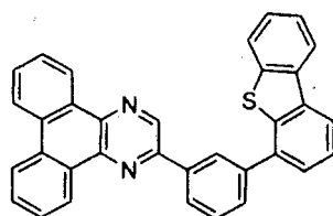
2mDBTPDBq-II
