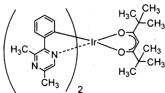
Ir(mppr-Me) 2 (dpm)
