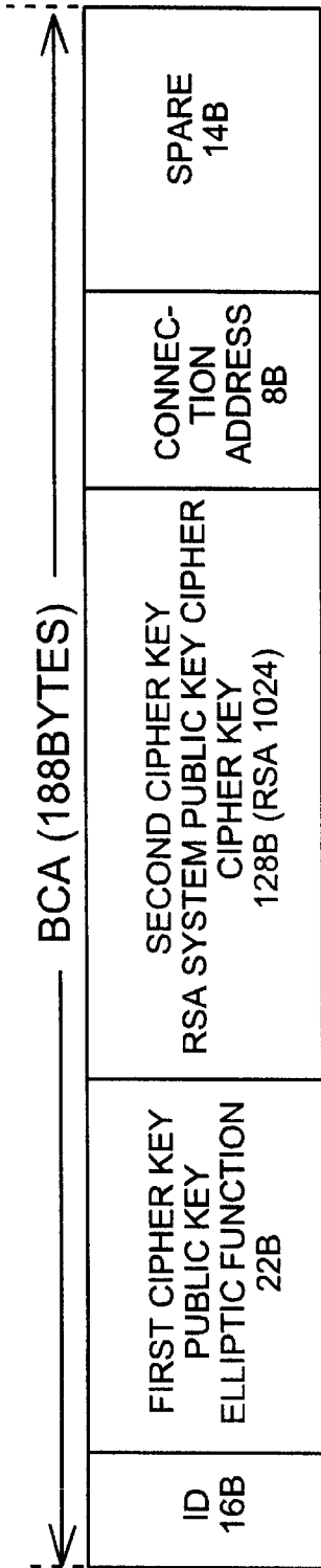
FIG. 7A
