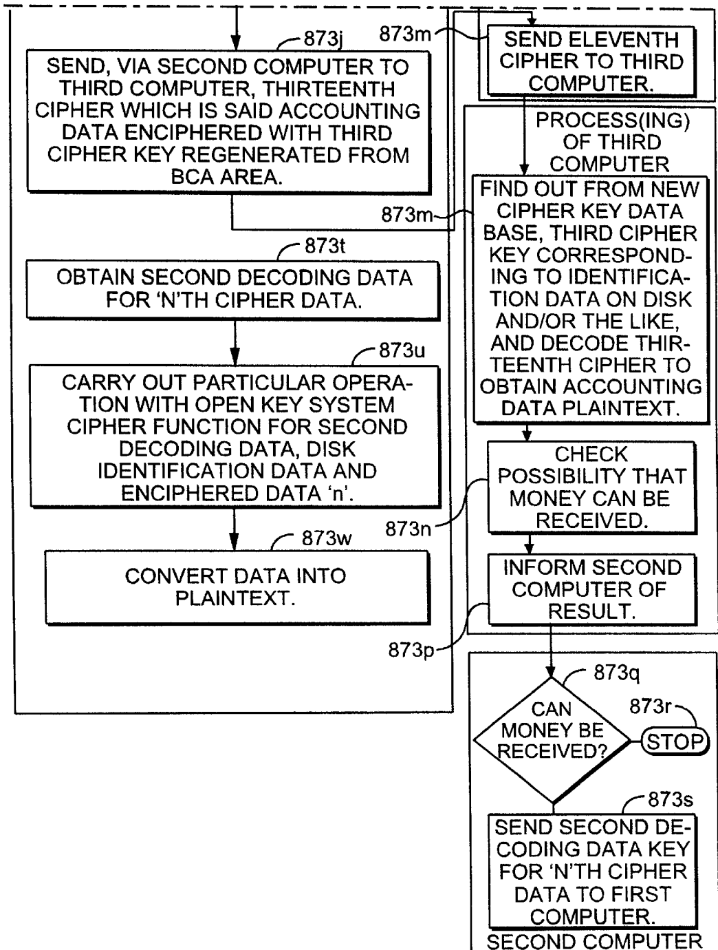
FIG. 23B
