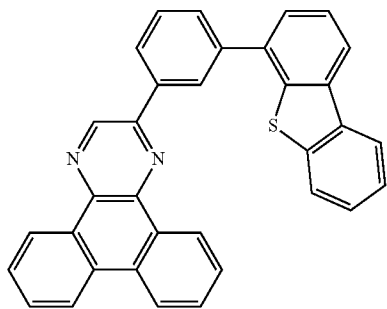
2mDBTPDBq-11
