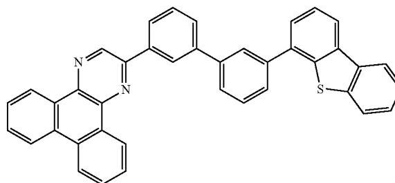
2mDBTPDBq-II
