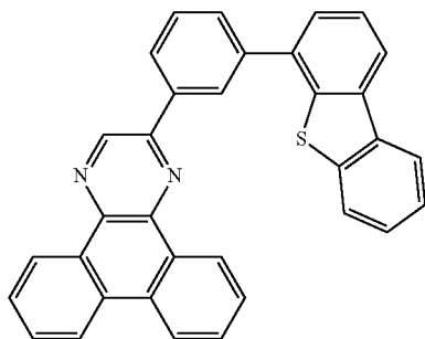
2mDBTPDBq-11
