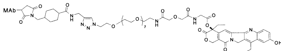
MAb-CL1-SN-38
