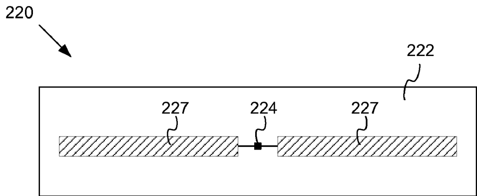
RFID TAG
