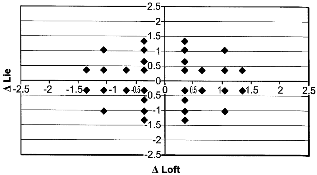
Loft / Lie Orientations (1°, 1/2°)
