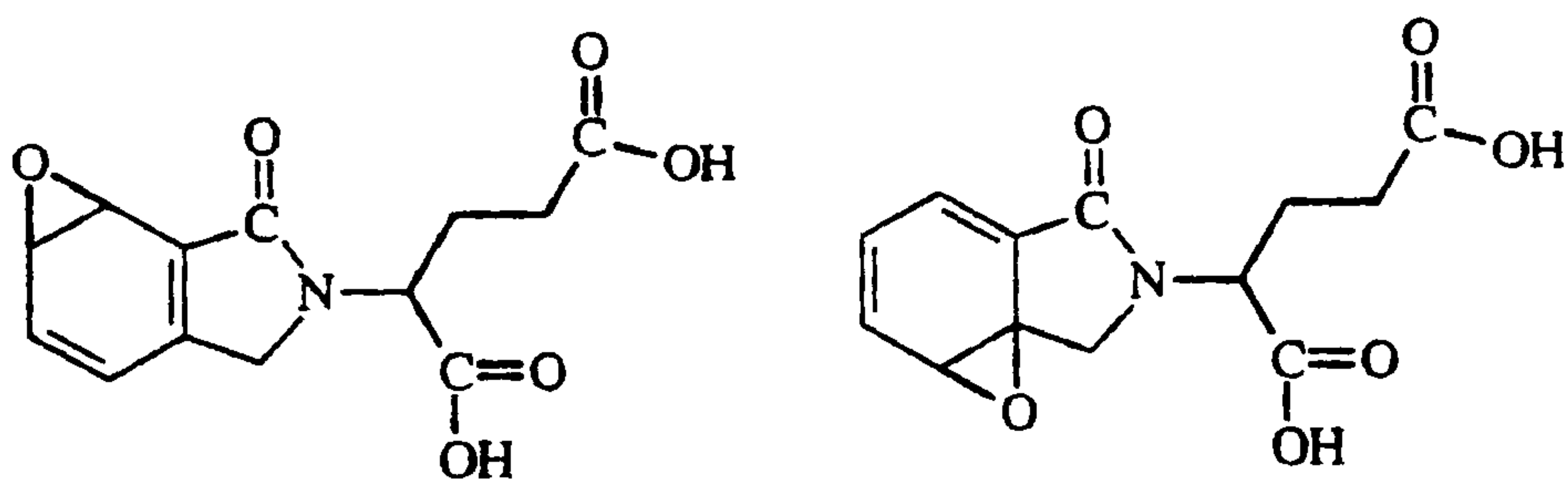
Epoxides of EM 138
