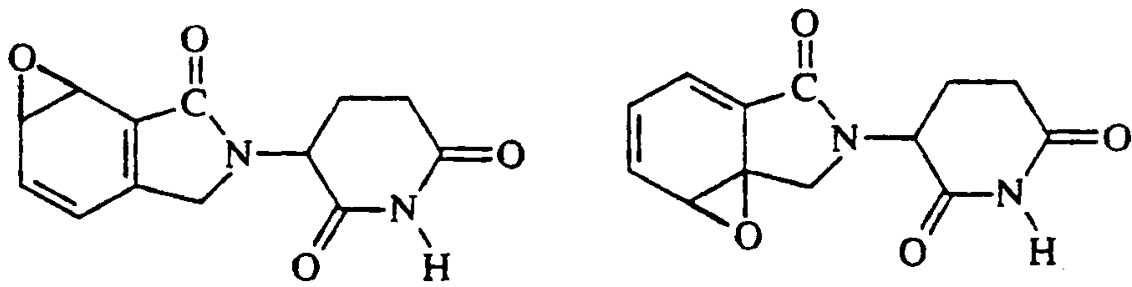
Epoxides of EM 12
