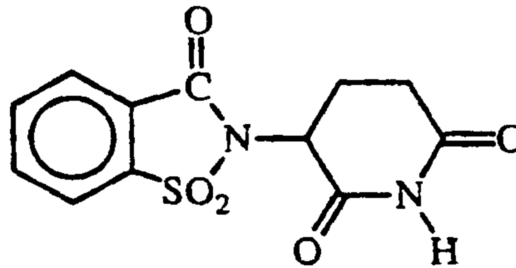
supidimide.
