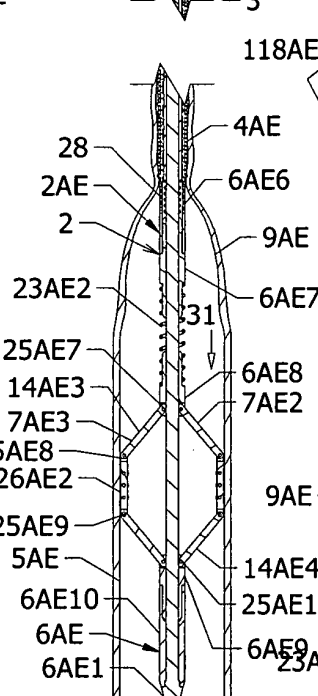
Fig. 98 SECTION AU-AU
