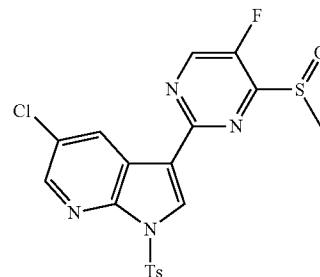
5-chloro-3-(5-fluoro-4-(methylsulfinyl)pyrimidin-2-yl)-1-tosyl-1H-pyrrolo[2,3-b]pyridine (1a)
