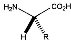
L- \alpha -amino acids
