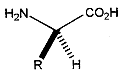
D- \alpha -amino acids
