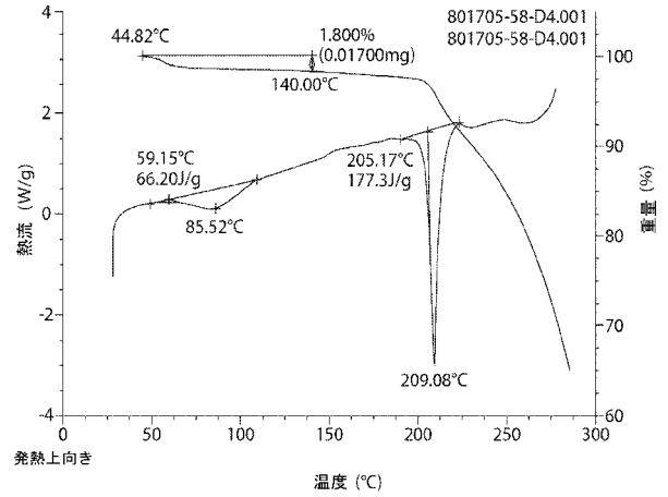
形態4のDSC及びTGAプロファイル
