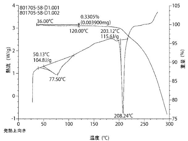
形態5のDSC及びTGAプロファイル
