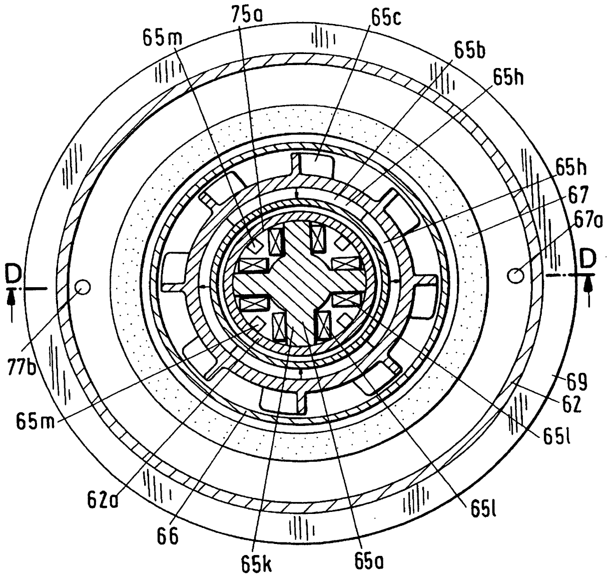
Fig.18 C-C
